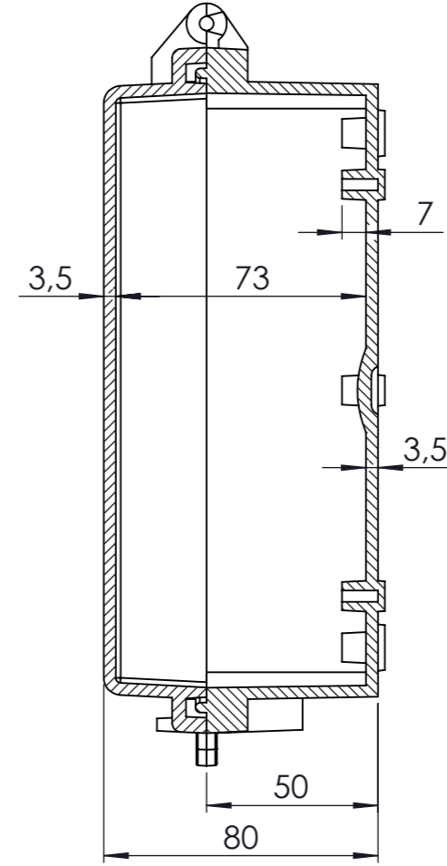
KESIT A-A
